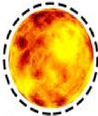
Sun
