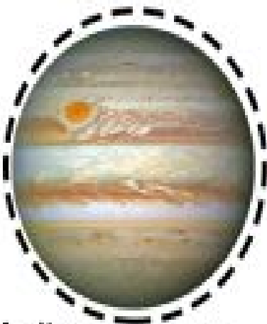
Jupiter
